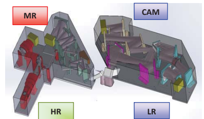
中間赤外線観測装置SMI光学配置
