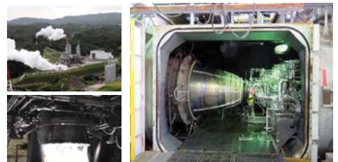
LE-5B-3エンジン燃焼試験
