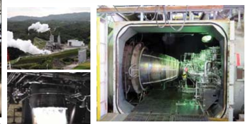
LE-5B-3エンジン燃焼試験
