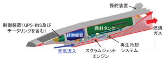
エアブリーザの飛行実証機の概略図
