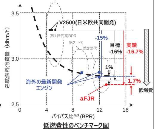
低燃費性のベンチマーク図
