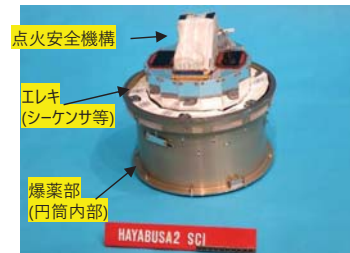
開発した衝突装置(分離機構除く) 分離機構によりスピン分離する
