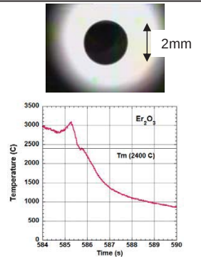
左上: ISS静電浮遊炉内で浮遊する酸化エルビウム融体(中央の白円部分) 右上: 真球となり浮遊する同融体(中央の黒円部分) 右: 同融体の加熱履歴。3,000℃以上の超高温状態を達成した。
