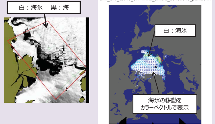
図7：(左)高解像度海水氷密度度 (右)海水移動ベクトル
