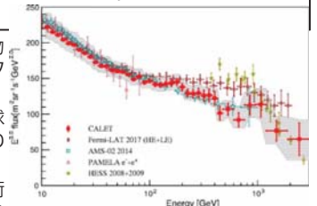
↑10GeV~3TeV電子・陽電子エネルギースペクトル(赤点)。宇宙線の主要成分の一つである電子成分(微量の陽電子成分を含む)については、これまで高エネルギー領域(GeV~TeV以上)での観測精度が不足していた。
