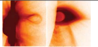
“教科書”的な噴出とカスプ構造発達をX線撮像・EUV分光診断(9/10フレア)
