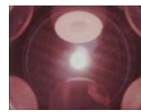
左上: ISS静電浮遊炉内で浮遊する酸化エルビウム融体(中央の白円部分) 右上: 真球となり浮遊する同融体(中央の黒円部分) 右: 同融体の加熱履歴。3,000℃以上の超高温状態を達成した。
