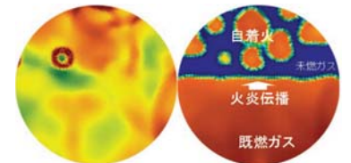
ノック(異常自着火)発生時の筒内圧力分布(左)と温度分布(右)
