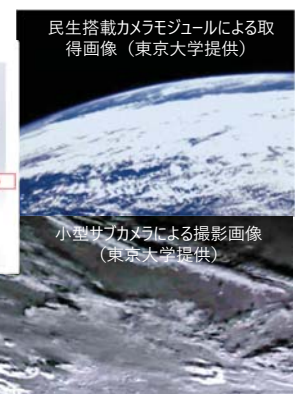
サイズ：116mm×116mm×346mm（アンテナ部除く） 重量：約3.2kg
