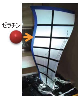
中空CFRPブレードの耐衝撃性試験
