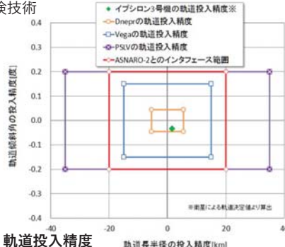
3号機打上げ(H30.1.18) / 軌道投入精度
