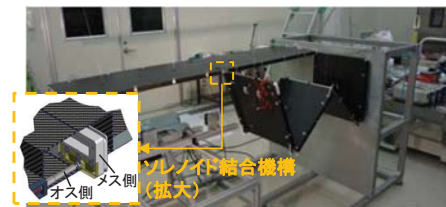
展開・結合機構の地上試験の様子
