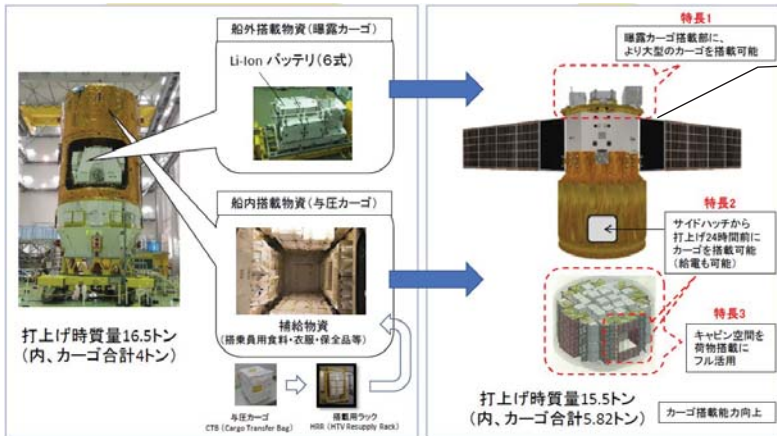
物資搭載効率の向上(HTVとの比較)
