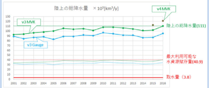
図6： GSMaPによる陸上総降水量の長期変動データ
