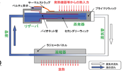
ループヒートパイプ（LHP）の構成・動作原理
