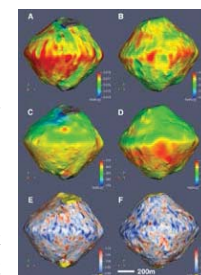
②関連図 リュウグウの形状モデルに投影したNIRS 3スペクトルの特徴。左側は西半球、右側は東半球を示す。A, Bは2.0 μmの反射率。C, DはNIRS 3による表面温度。E, Fは2.72 μm吸収強度。
