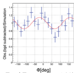
図1：今回のASTRO-H SGDによる観測で得られたかに星雲からの偏光ガンマ線エミッションカーブ
