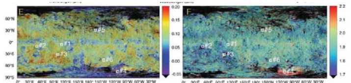
③関連図 6地点をスペクトルの傾き分布(E)と0.55μmでの反射強度分布(F)にプロット。
