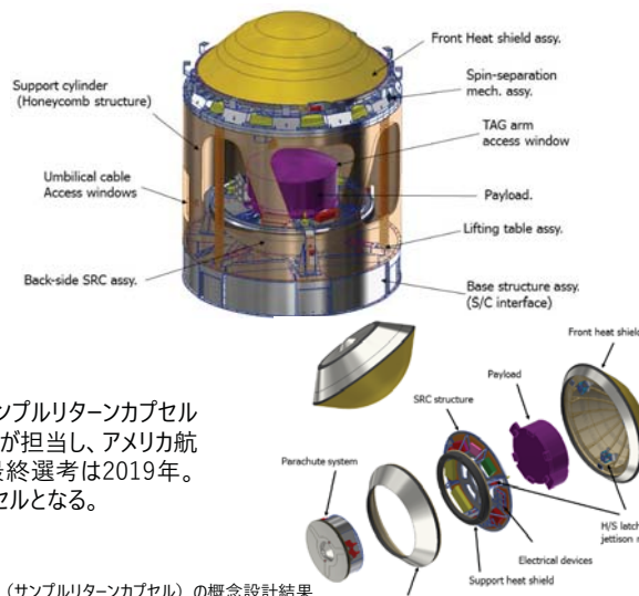
CAESAR-SRC（サンプルリターンカプセル）の概念設計結果
